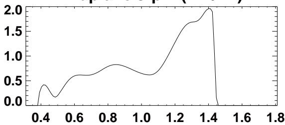
Midplane poloidal flux (Wb)
