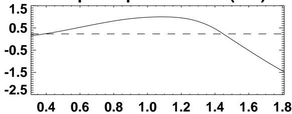
Midplane poloidal flux (Wb)
