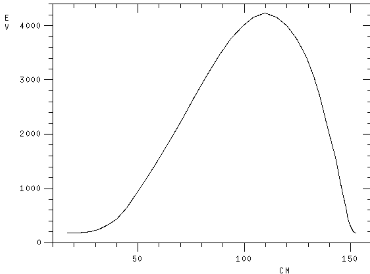
ION TEMPERATURE (TI) VS MIDPLANE RADII (RMAJM)
