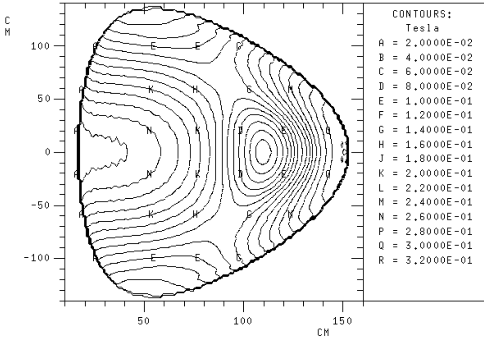
mod(Bpol) CONTOUR PLOT VS R & Y
